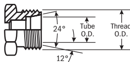
Male 24° Cone
