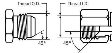
SAE 45° Flare Male (MS)
